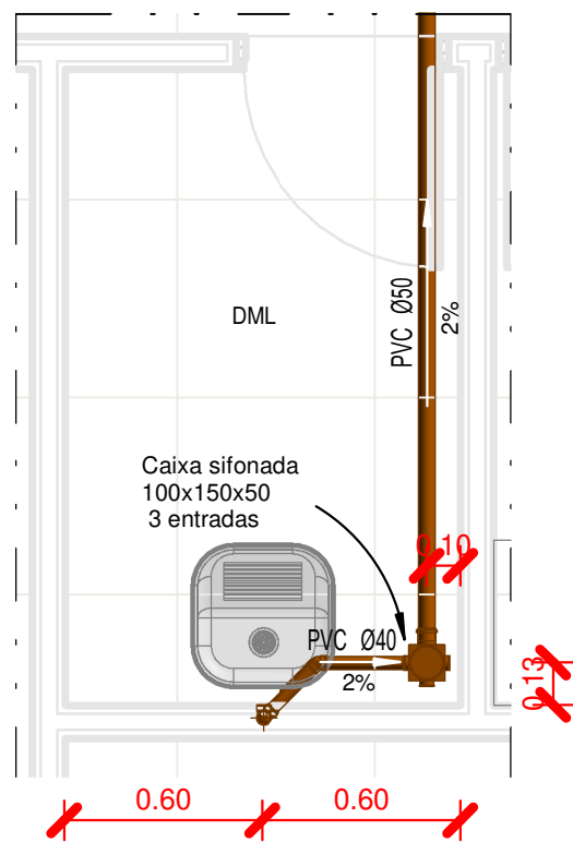
DETALHE 04 - ESGOTO
