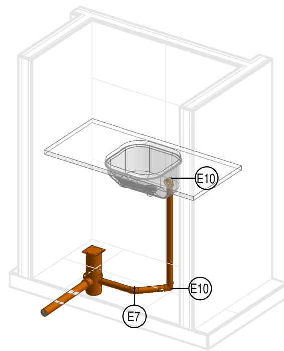
PERSPECTIVA 04 - ESGOTO
