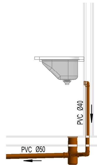
VISTA 04 - ESGOTO
